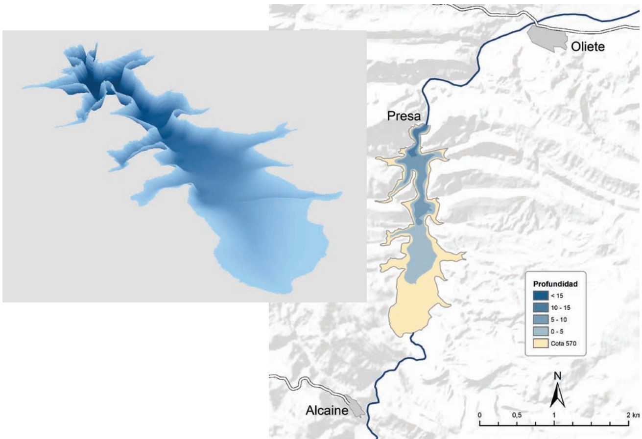
Figura 4. Batimetría del embalse de Cueva Foradada
