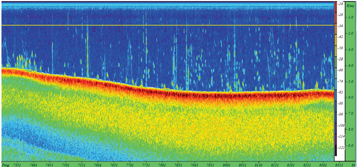
Figura 13. Ejemplo de ecograma en una de las zonas parcialmente sometidas a burbujeo en el embalse de Cueva Foradada
