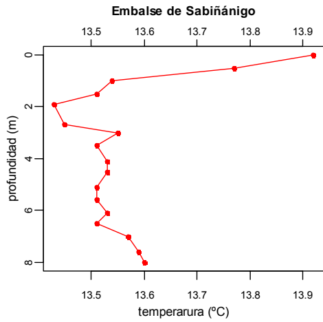
GRÁFICO 1 PERFILES FÍSICO-QUÍMICOS DEL EMBALSE DE SABIÑÁNIGO
