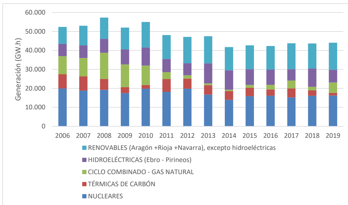
Figura 03.27. Evolución de la generación eléctrica con distintas tecnologías en la demarcación hidrográfica del Ebro (2006-2016). Fuente: REE
