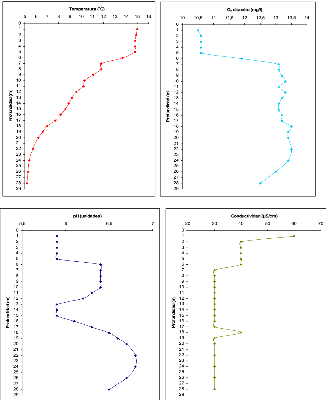
GRÁFICO 1 PERFILES FÍSICO-QUÍMICOS DEL ESTANY
